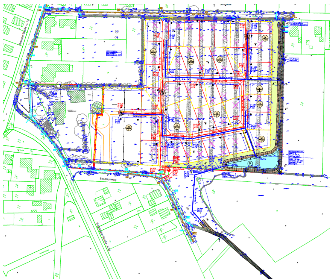
Abb.: Entwässerungsplan, Stand: 12.09.2018, Quelle: Thalen Consult GmbH
